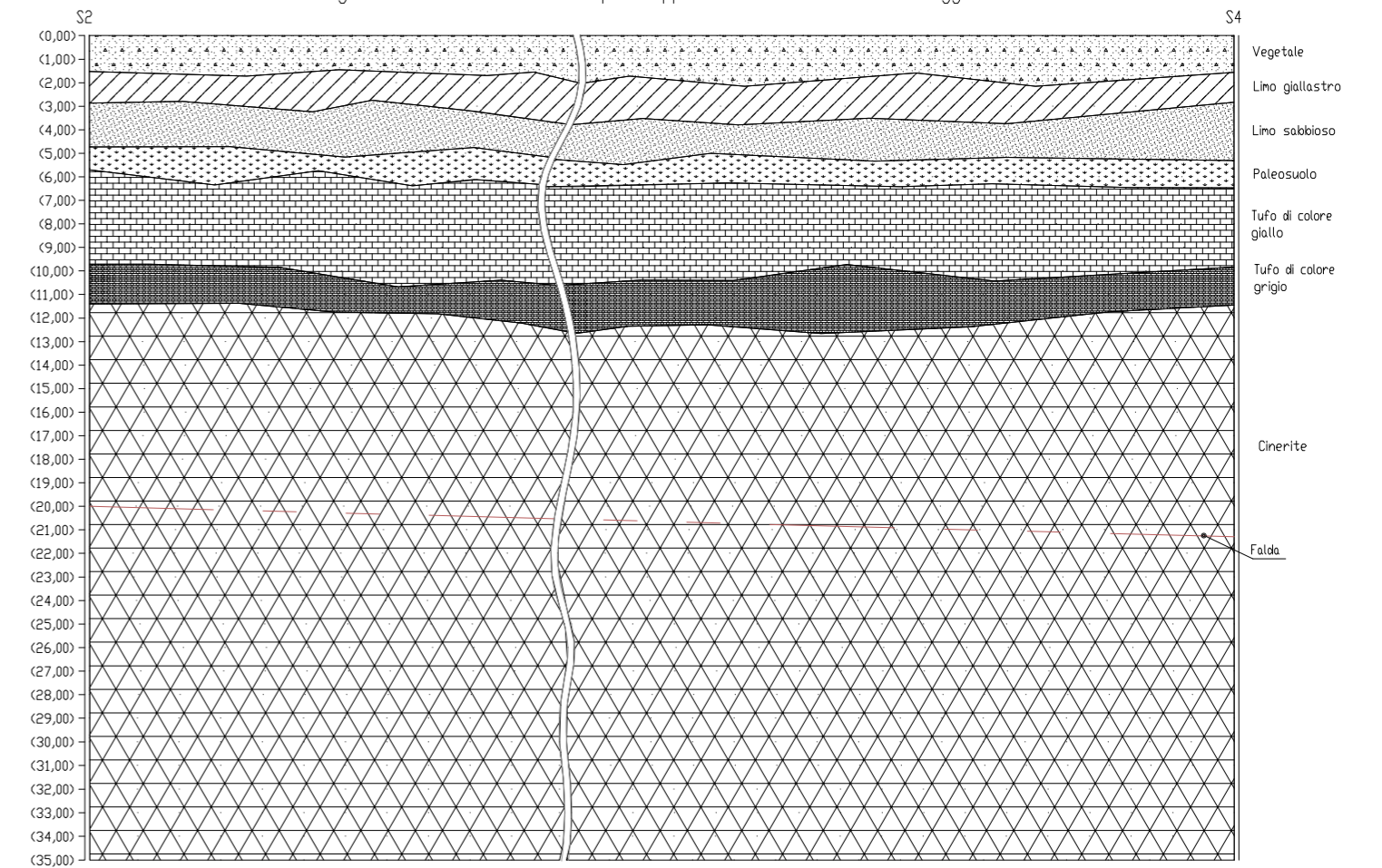
Sezione stratigrafica schematica ricavata per supposta continuità fra i sondaggi S4 - S3
