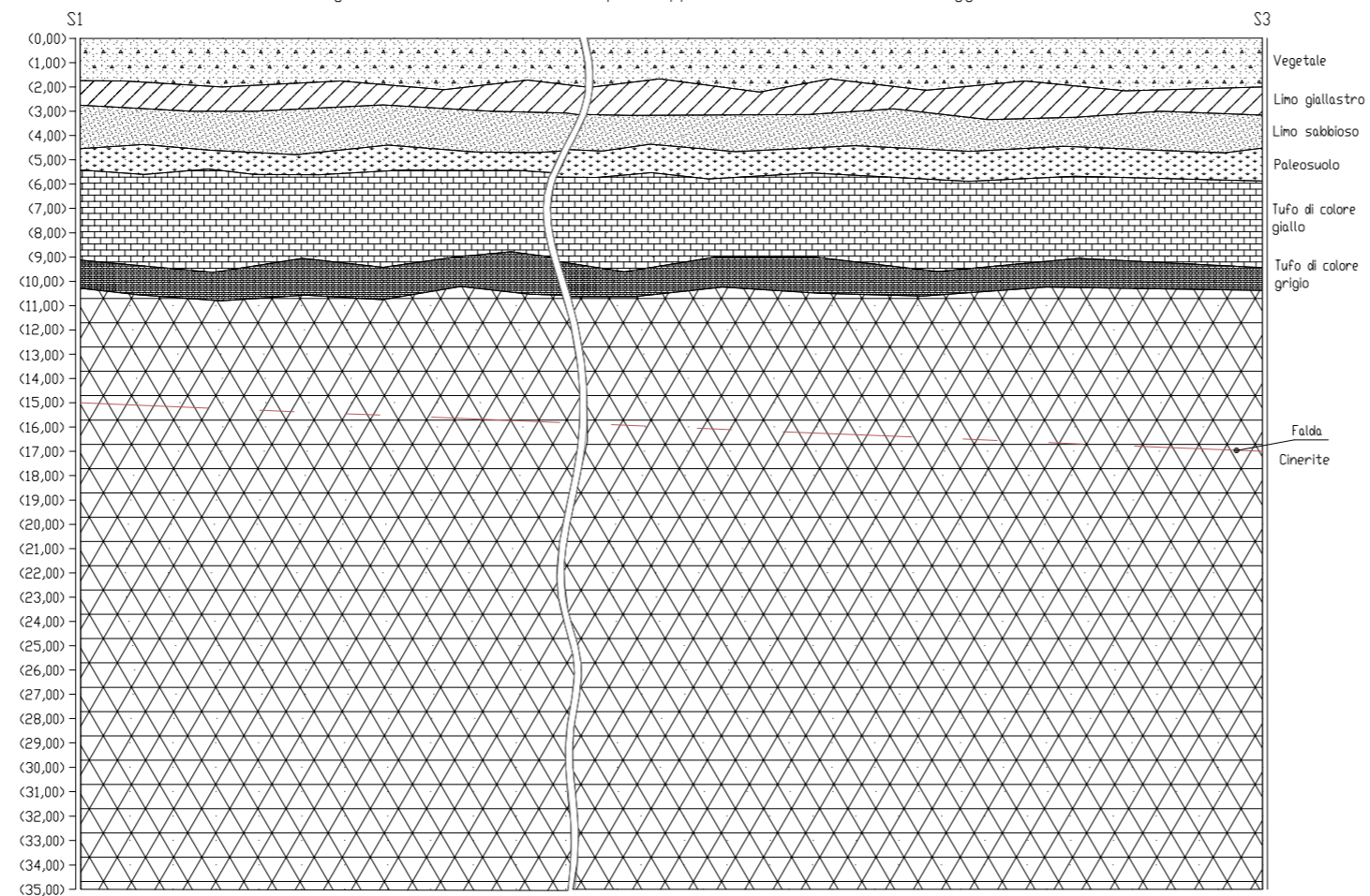
Sezione stratigrafica schematica ricavata per supposta continuità fra i sondaggi S2 - S3
